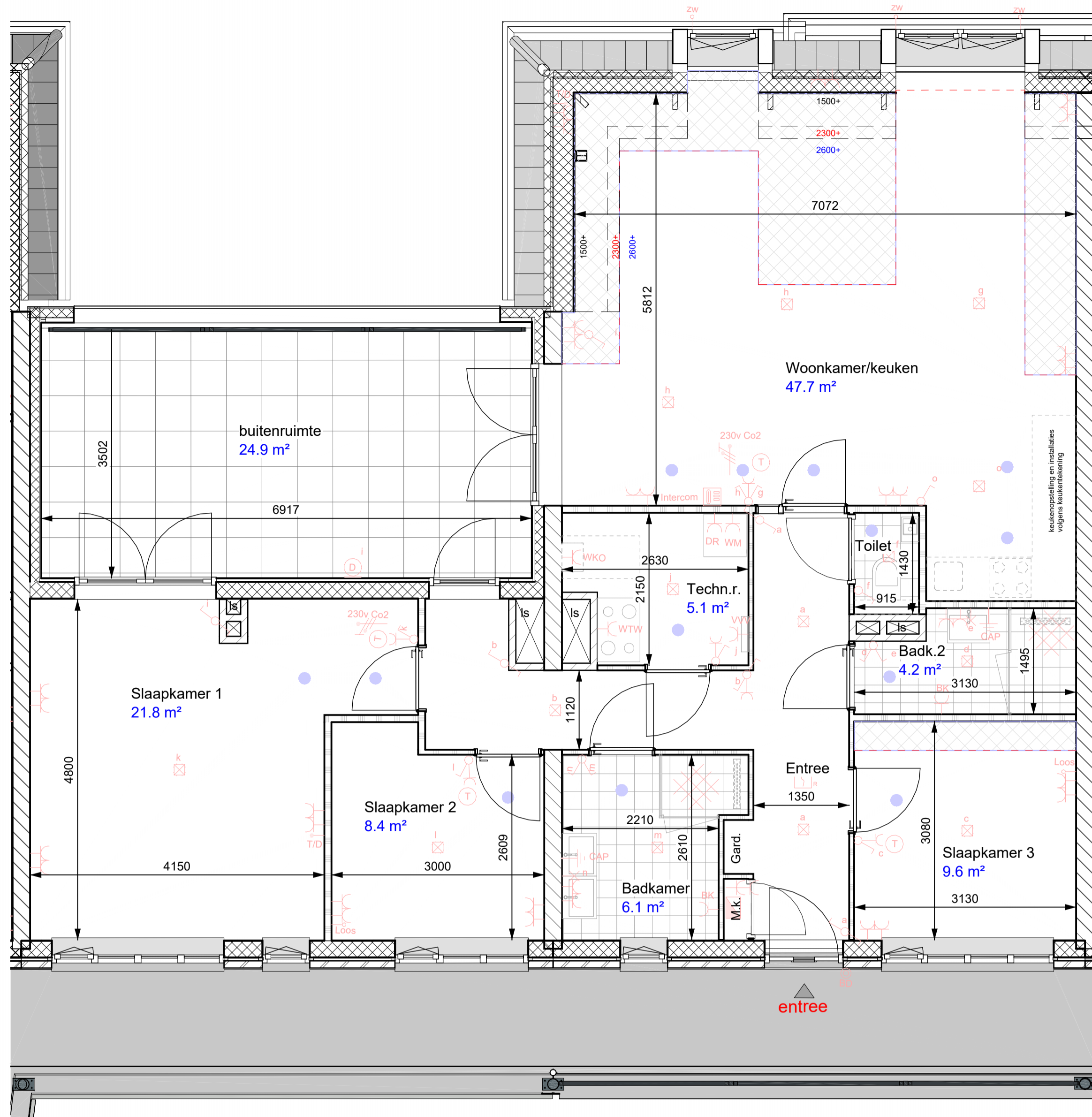
Plattegrond
